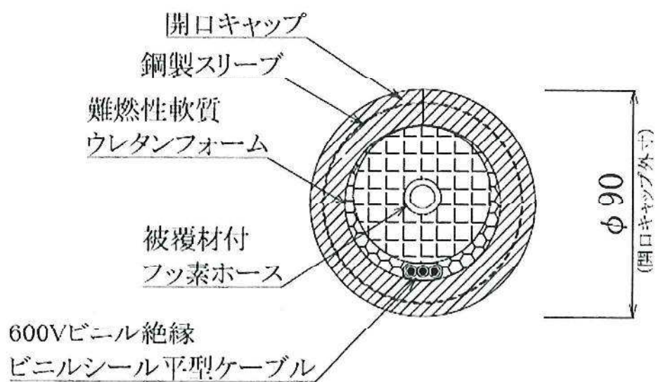
立断面図
