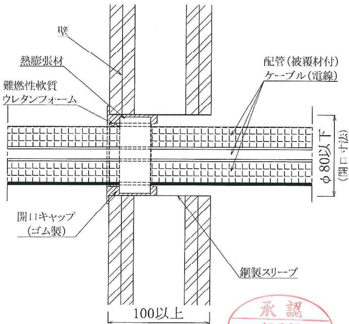
図2 施工図例
