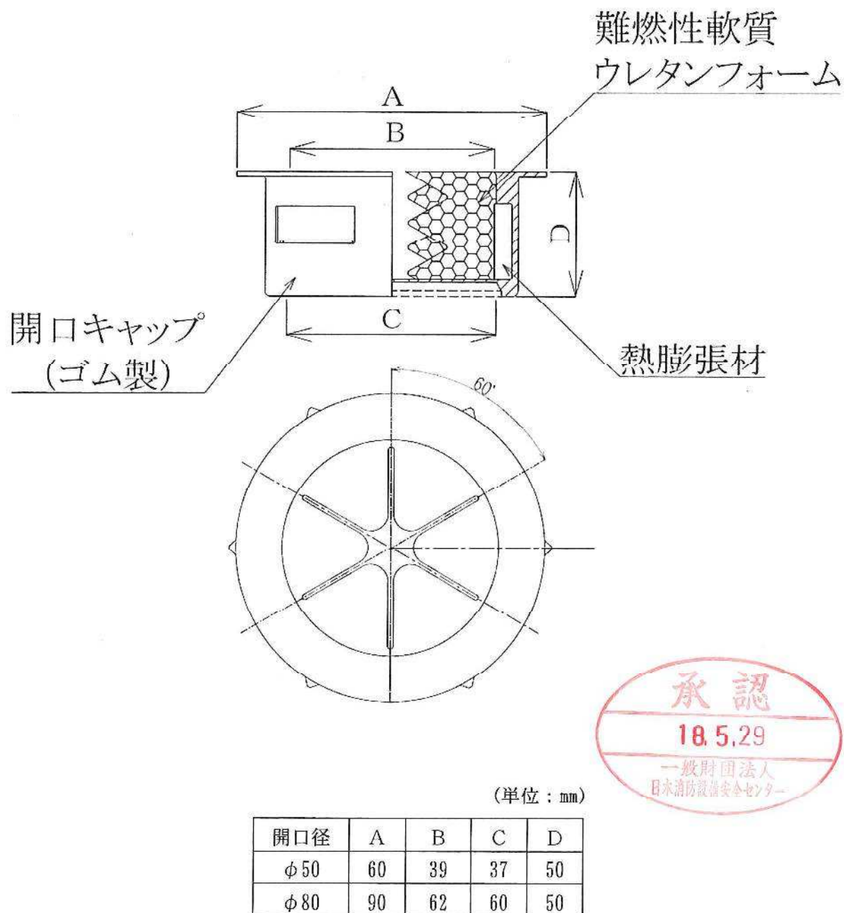
図1 開口キャップ（熱膨張材、ウレタンフォーム組込み）構造、種類及び寸法
